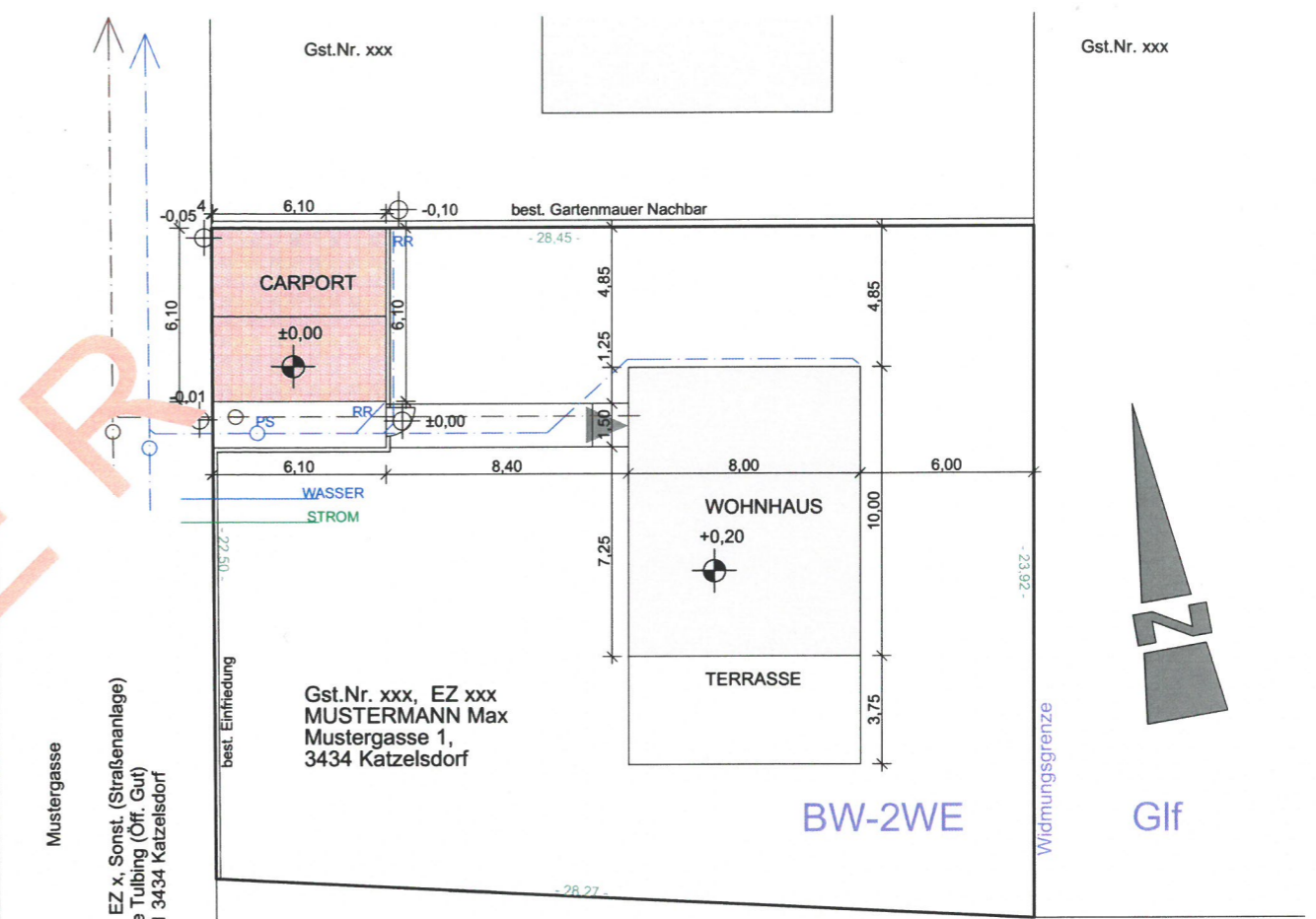
LAGEPLAN 1 : 250 rechtlich gesicherte Grenzen/Grenzkataster
